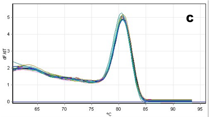
Fig S2A: Melting curves for the reference genes : (A) ACTB , (B) TUBB , (C) RPL12 , and (D) SRP54 .
