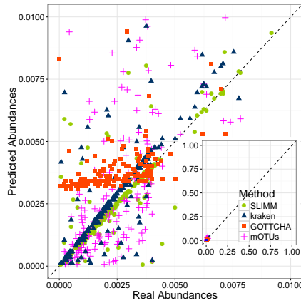
(d) random-0500-1000
