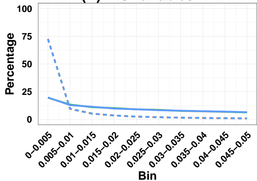
(D) 8 variables
